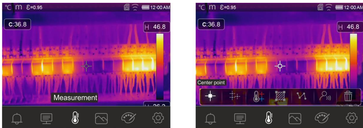
Fig. 34: Menú Medida
