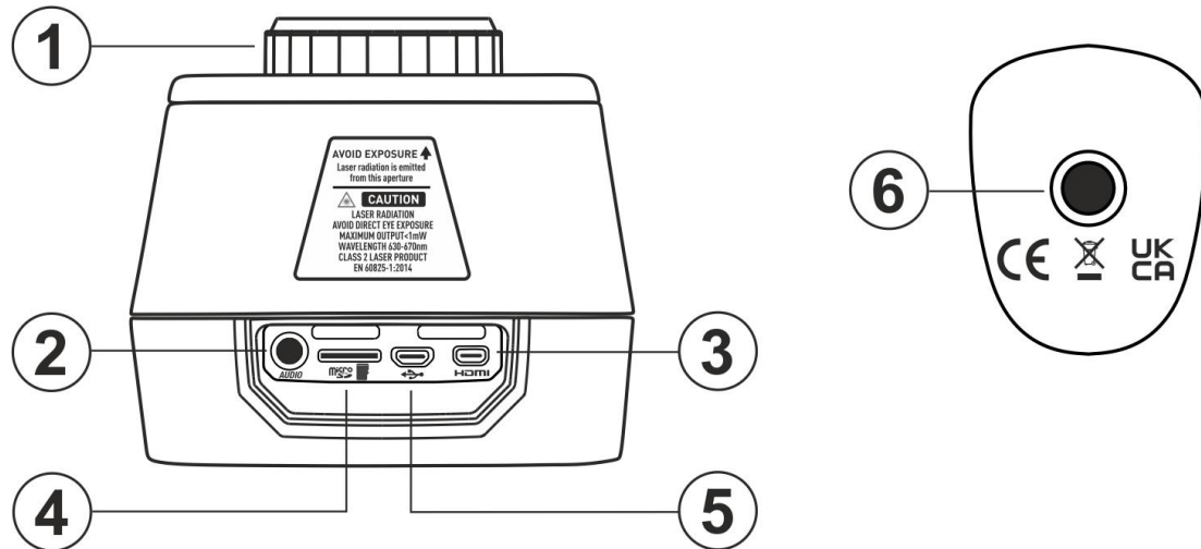
Fig. 4: Descripción parte superior y inferior del instrumento
