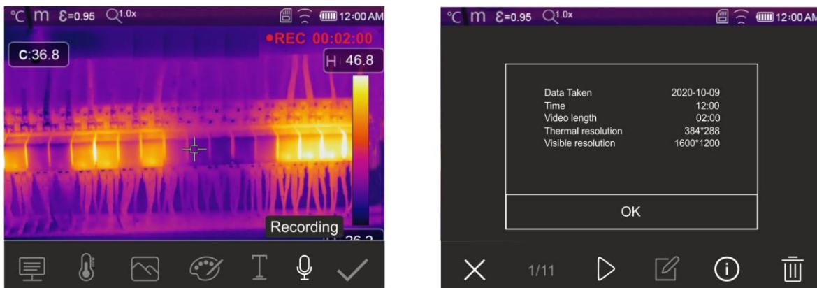
Fig. 51: Registro vídeo IR
