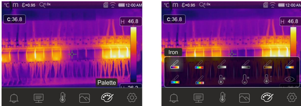
Fig. 40: Selección paletas colores y funciones isotermas
