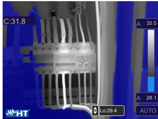
Fig. 42: Selección isoterma Alarm low Temp
