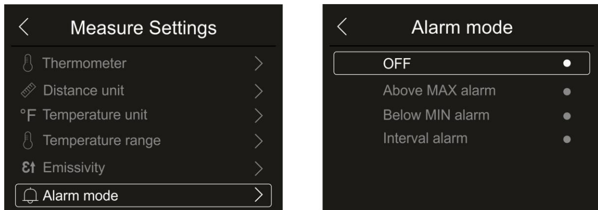
Fig. 29: Menú activación umbrales de alarma sobre la medida
