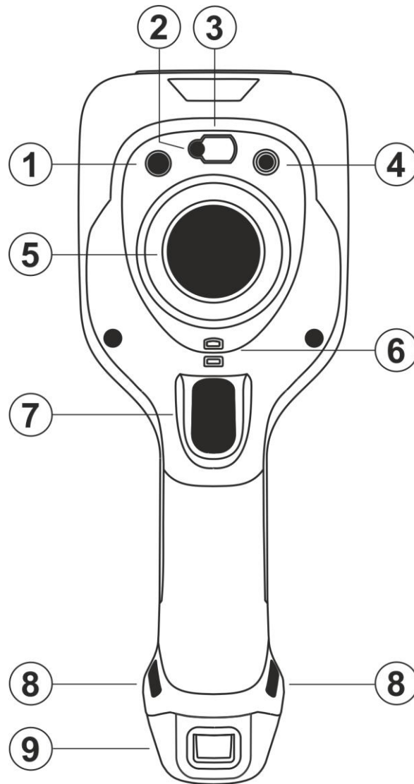
Fig. 2: Descripción delantera del instrumento
