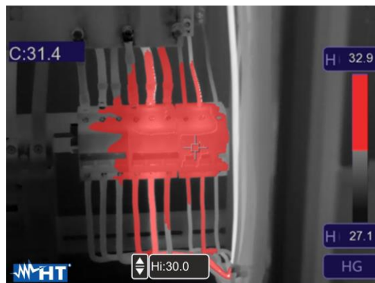
Fig. 41: Selección isoterma Alarm high Temp
