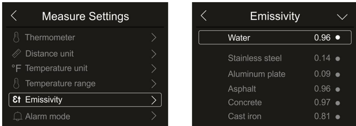
Fig. 28: Menú configuración Emisividad
