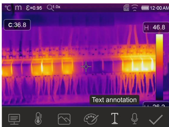
Fig. 49: Inserción nota de texto en la imagen
