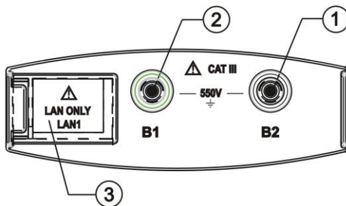
Fig. 2: Descripción de los terminales de entrada del instrumento
