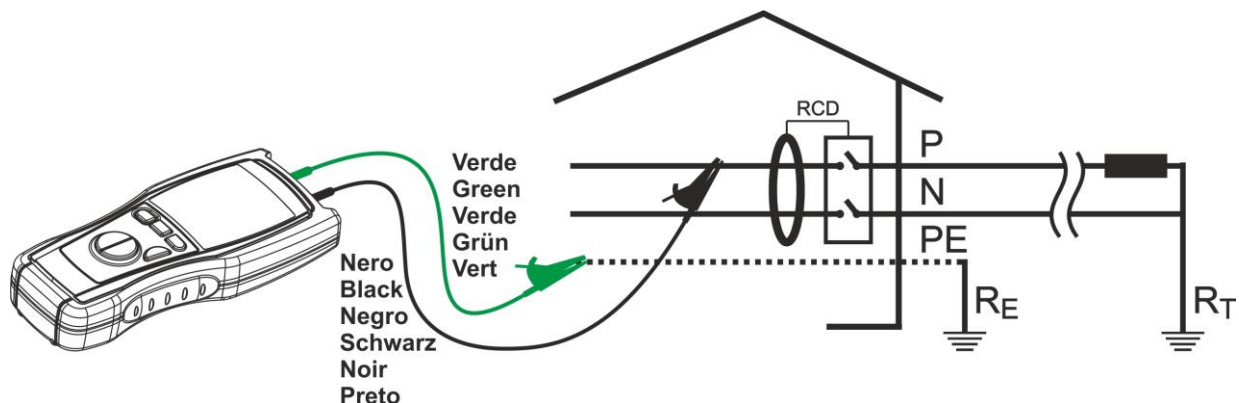
Fig. 11: Conexión de los terminales del instrumento
