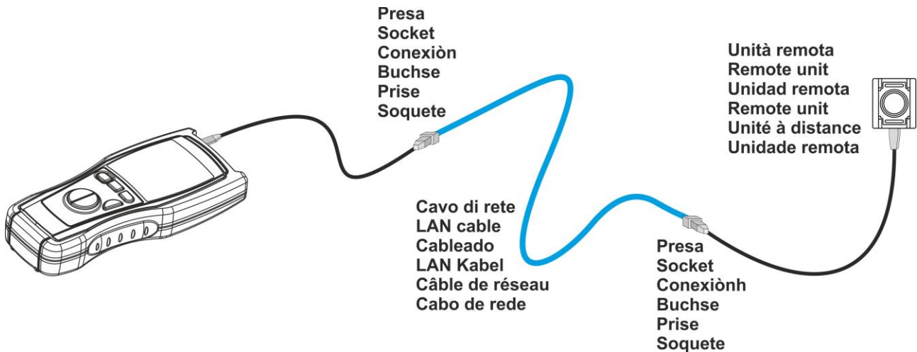
Fig. 8: Conexión de las puntas de prueba del instrumento
