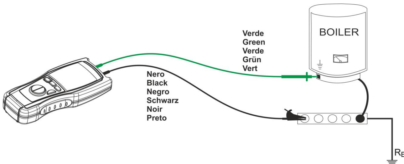
Fig. 9: Conexión de las puntas de prueba del instrumento en continuidad \Omega 0.2A
