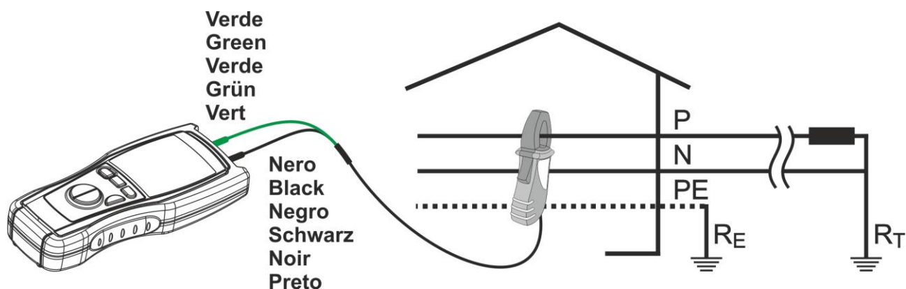
Fig. 4: Conexión de las puntas de prueba del instrumento
