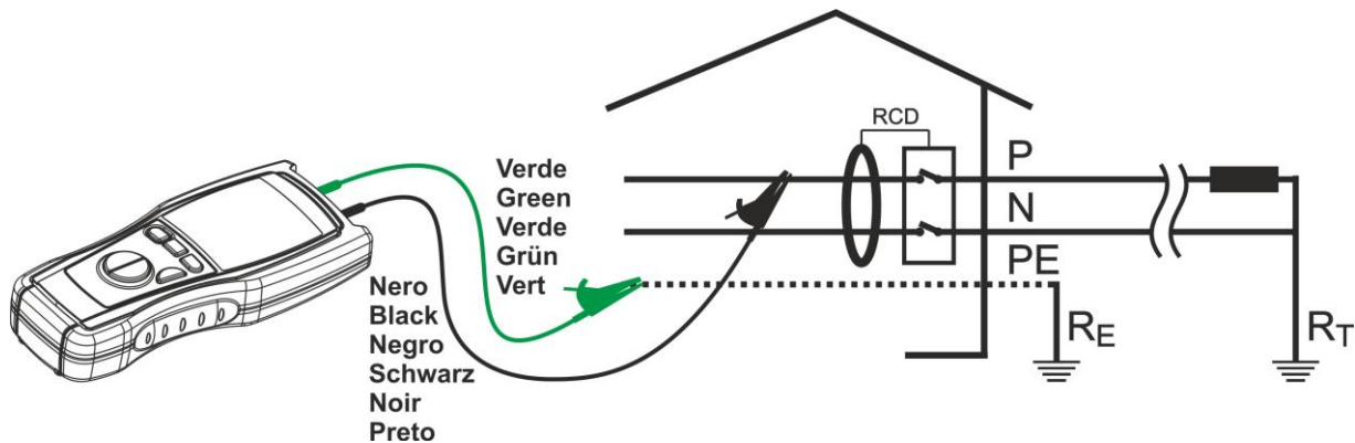
Fig. 12: Conexión de los terminales del instrumento
