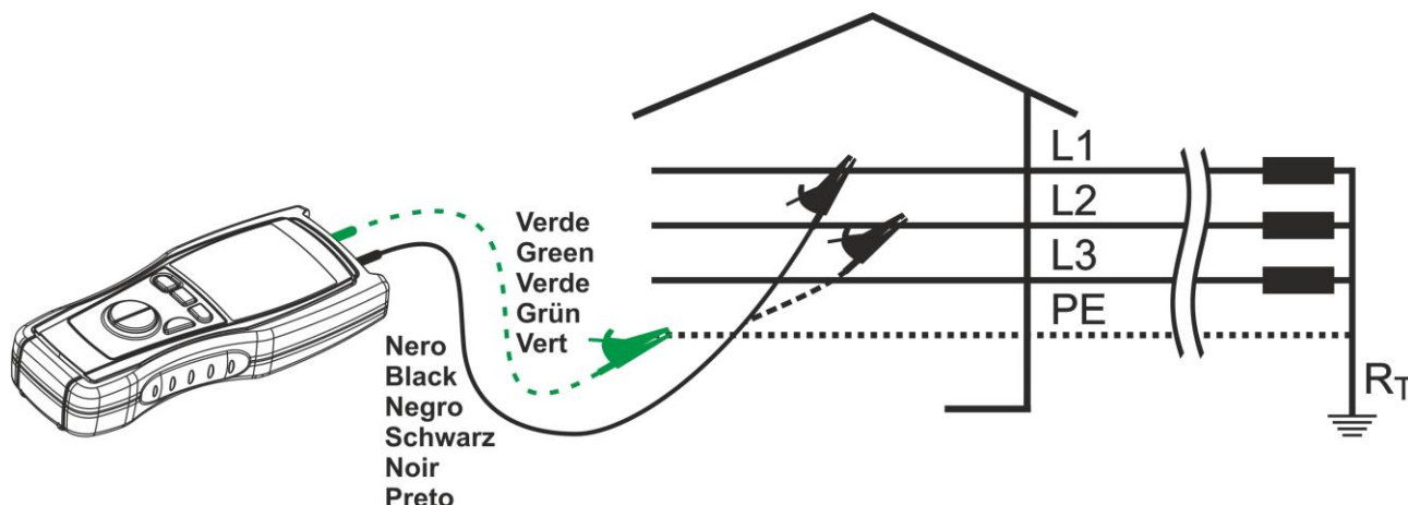
Fig. 7: Conexión de las puntas de prueba del instrumento
