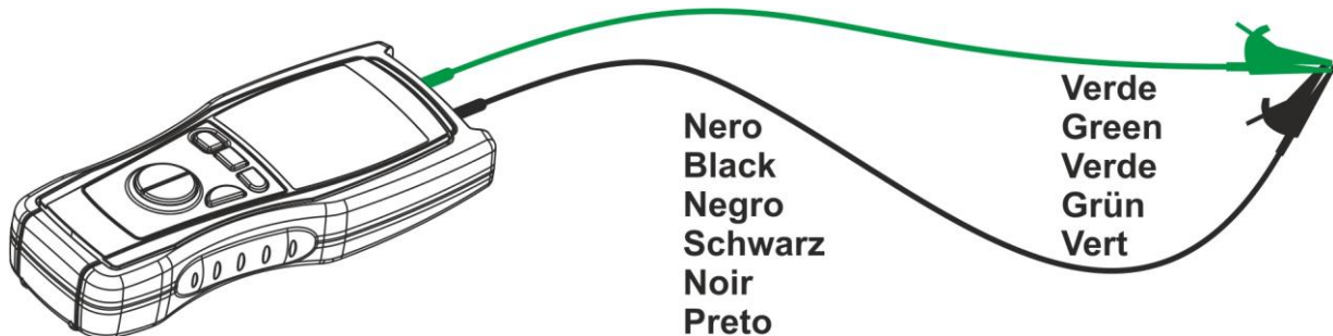
Fig. 10: Conexión de los terminales durante el procedimiento de calibración
