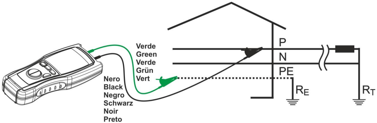
Fig. 3: Conexión de las puntas de prueba del instrumento en V \approx Hz
