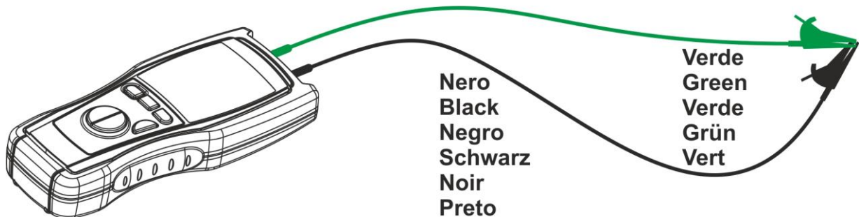
Fig. 6: Conexión de los terminales durante el procedimiento de calibración
