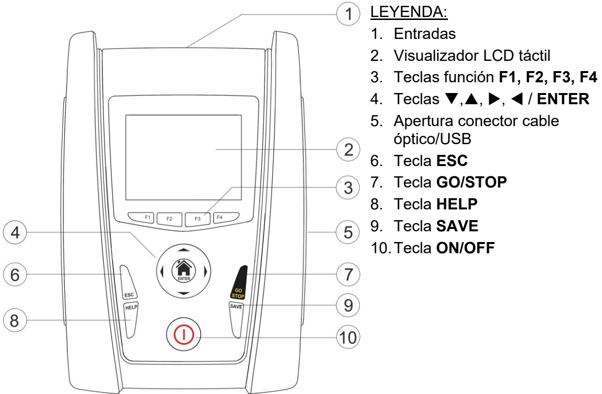
Fig. 1: Descripción parte frontal del instrumento
