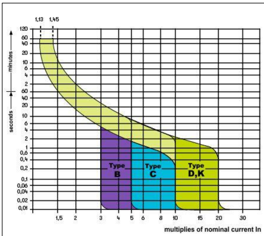
Fig. 46: Ejemplo de curvas de intevento de protección magnetotérmica (MCB)
