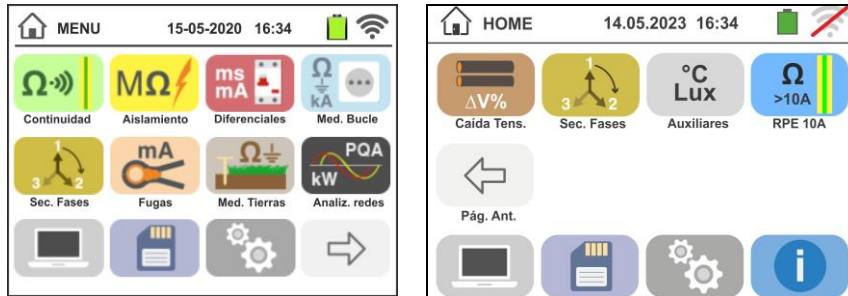
Fig. 5: Menú general instrumento
