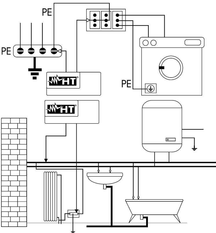
Fig. 44: Ejemplos de medidas de continuidad de los conductores
