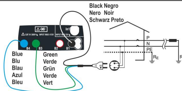
Fig. 18: Medida P-N/P-PE en instalaciones monofásica 230V mediante toma shuko
