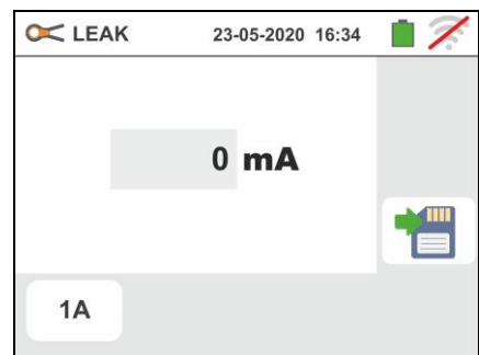
Fig. 27: Medida directa de la corriente de fuga en instalaciones trifásicas
