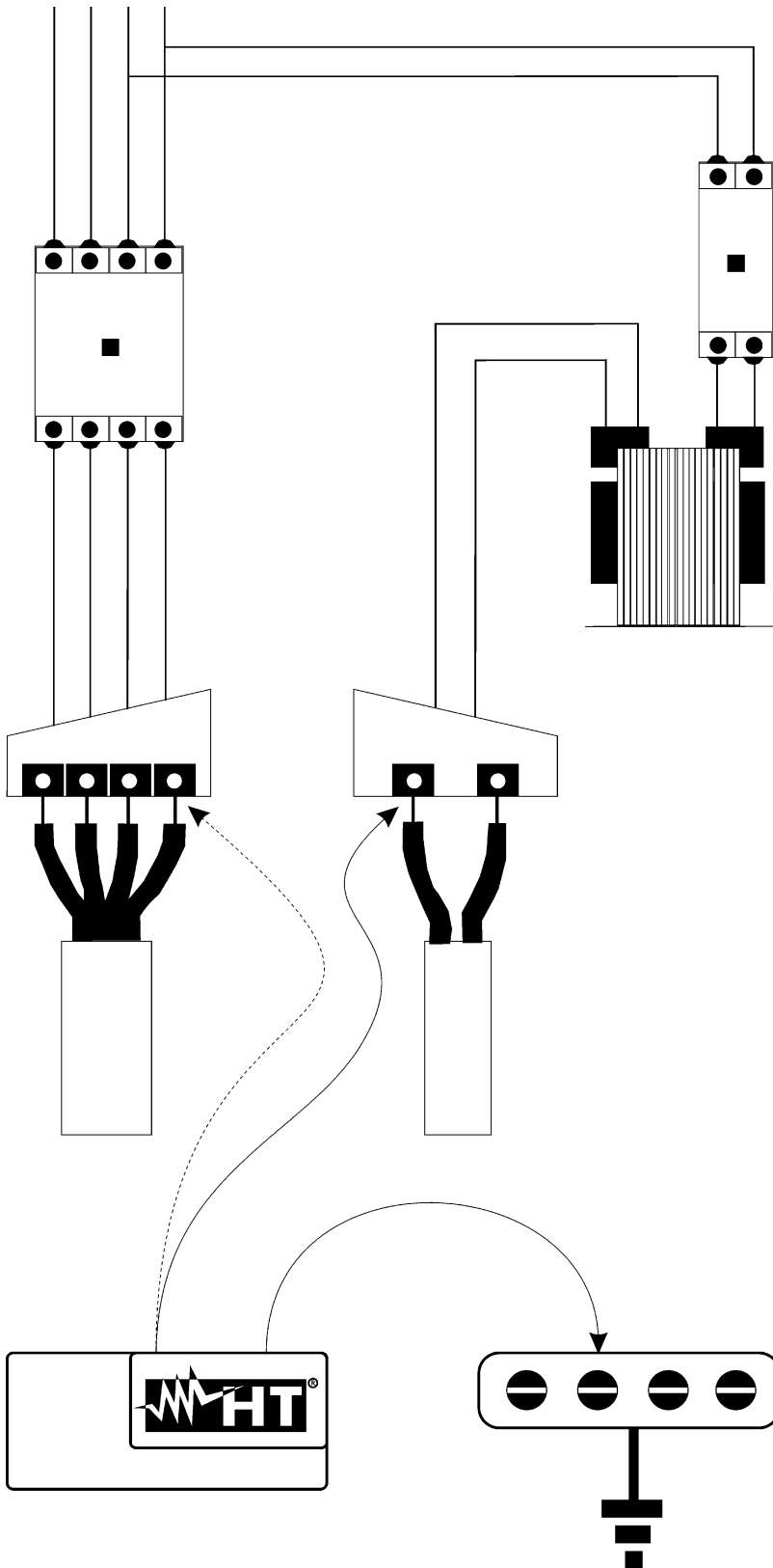
Fig. 45: medidas de separación entre circuitos en una instalación
