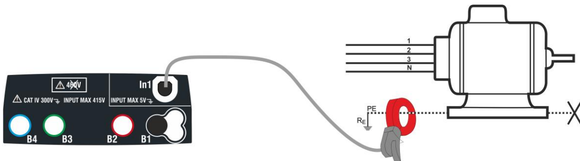
Fig. 27: Medida directa de la corriente de fuga en instalaciones trifásicas
