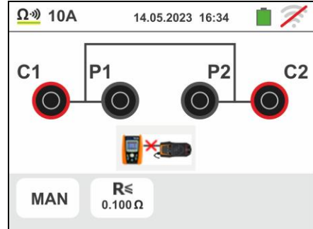
Fig. 36: Medida Continuidad de conductores de protección con accesorio EQUITEST
