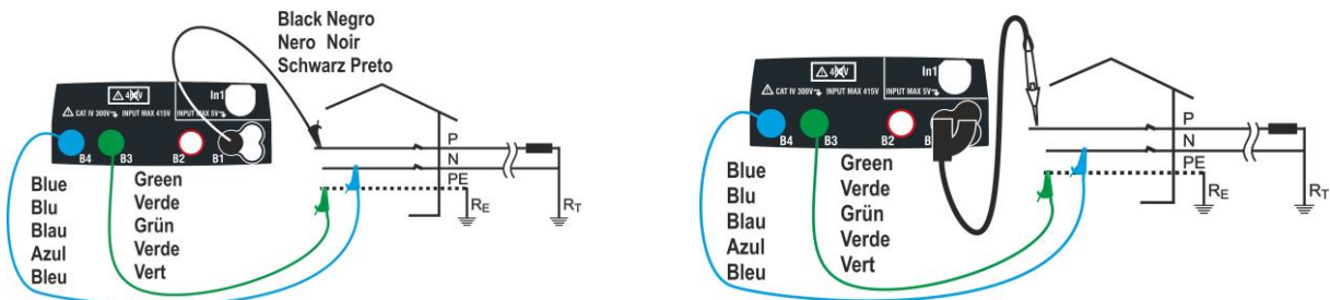
Fig. 19: Medida P-N/P-PE mono/bifásicas 230V con cables y punta remota
