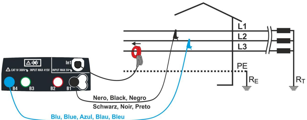
Fig. 38: Conexión para medida en sistema Trifásico equilibrado
