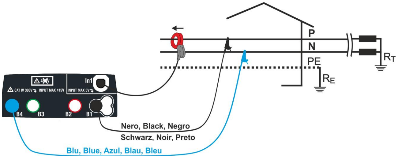
Fig. 37: Conexión para medida en sistema Monofásico
