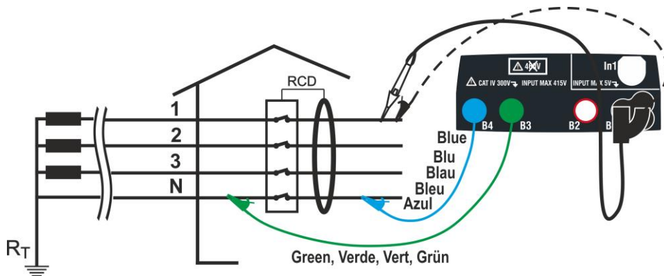
Fig. 15: Conexión 400V+ N (no PE) con cables y punta remota
