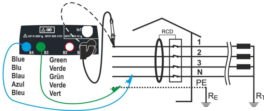
Fig. 14: Conexión en sistema trifásico 400V + N + PE con cables y punta remota
