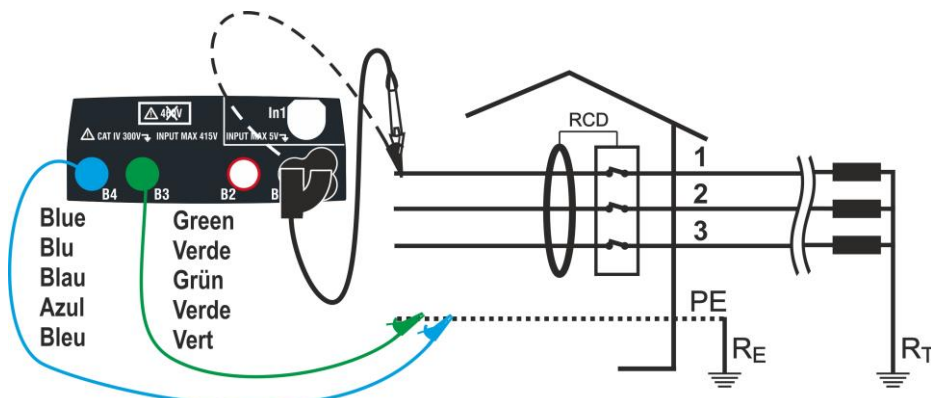
Fig. 16: Conexión en sistema trifásico 400V+ PE (no N) con cables y punta remota (no para RCD tipo B)
